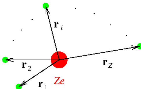
13.1. ábra. Atomi kordináták egy atommag körül.
