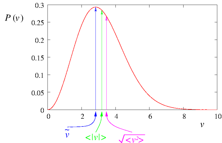
3.4. ábra. A Maxwell-féle sebességeloszlás. A sebesség legvalószínűbb ( \tilde{v} ), átlagos ( \langle |v| \rangle ), illetve a sebessénégyzet gyökének várható értéke \sqrt{\langle v^2 \rangle} .
