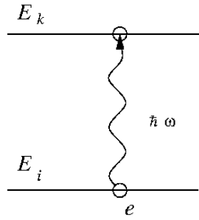
14.1. ábra. A fény okozta gerjesztés szemléltetése.
