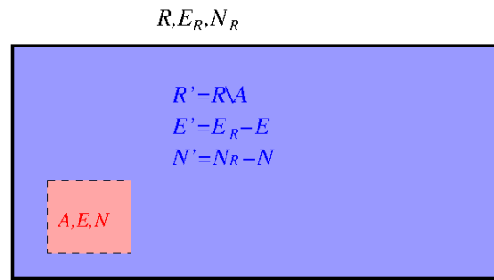
4.1. ábra. A nagykanonikus sokaság szemléltetése. A nagy R zárt rendszer része a kis A rendszer. Az A alrendszer hőt és részecskét is cserélhet az R' = R \setminus A rendszerrel.
