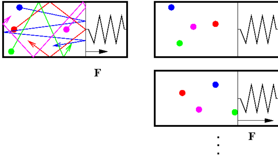
1.2. ábra. Az időátlag (balra) és a sokaságátlag (jobbra) szemléltetése. A jobb oldali falon mérjük a nyomást. Az időátlag során a T idő alatt létrejött ütközések impulzusváltásához szükséges erőt mérjük. Sokaságátlag során az össze mikroállapotot soravesszük megfelelő \rho(q, p) súllyal. Lesznek esetek, amikor egyetlen részecske sem lesz kölcsönhatásban a fallal ezek járuléka 0, azonban, amikor kontaktus van a fal és a részecske között, akkor a mikroszkópikus erőhatásoknak megfelelő erőjárulékot kapunk. Ezen mennyiségek átlagából kapjuk meg a nyomást.
