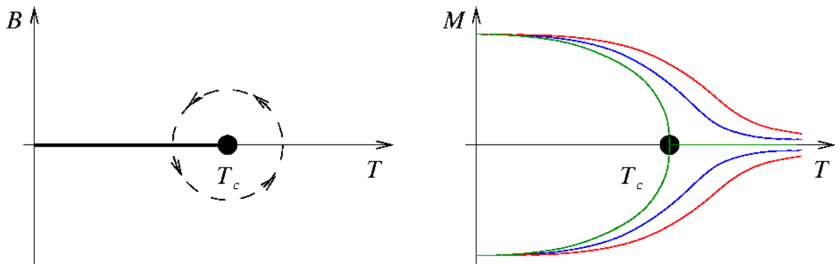
6.7. ábra. Ferromágneses fázisdiagram. Bal: B - T diagram. A kritikus pont kör-bejárható. Tehát hőmérséklet emelésével fázisátalakulás nélkül is át tudunk jutni a fázishatáron. Jobb: M - T diagramm különböző külső mágneses tér mellett, zöld zérus, kék kicsi, piros nagyobb külső mágneses térhez tartozó fázishatárok.
